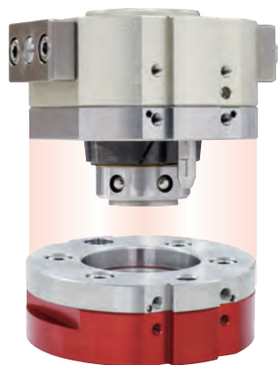
ツールアダプタ model SMR0120-T
